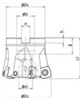
● fig.1 クーラント穴付き Through coolant hole (カッタ径φDc ≤ φ100)
