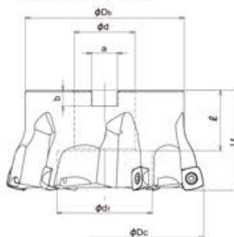
● fig.2 クーラント穴なし Without coolant hole (カッタ径φDc ≥ φ125)
